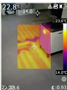
Het IR beeld als centrale rechthoek in het gewone visuele beeld als overlay. Opmerking: IR en VIS beeld vallen op het scherm NIET precies over elkaar heen hoewel dit op deze foto wel lijkt!
