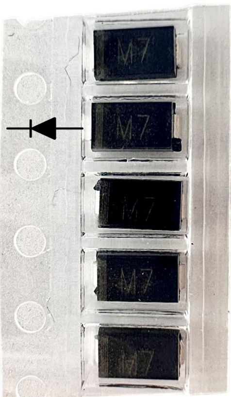
5x IN4007 rectifier diode D1-D5
